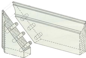
Assemblage par tourillons.
