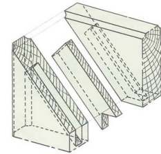
Cette fausse languette ne sort pas sur le champ extérieur.
