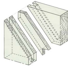
Assemblage par fausse languette.
