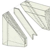
Fausse languette prise dans un placage épais.
